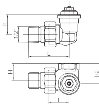
Fig. 9. Triaxe
