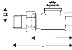
Fig. 7. Droit
